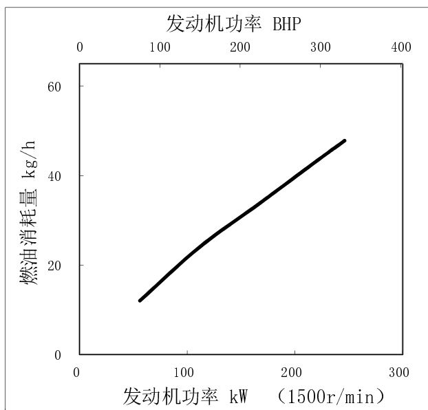
1500r/min主要性能参数
